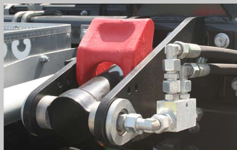
VERROUILLAGE HYDRAULIQUE AVANT
